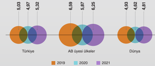
Türkiye, AB ve Dünya Ortalamasına Göre Kişi Başına Düşen Fosil Karbon Emisyon Miktarı (ton CO 2 )
