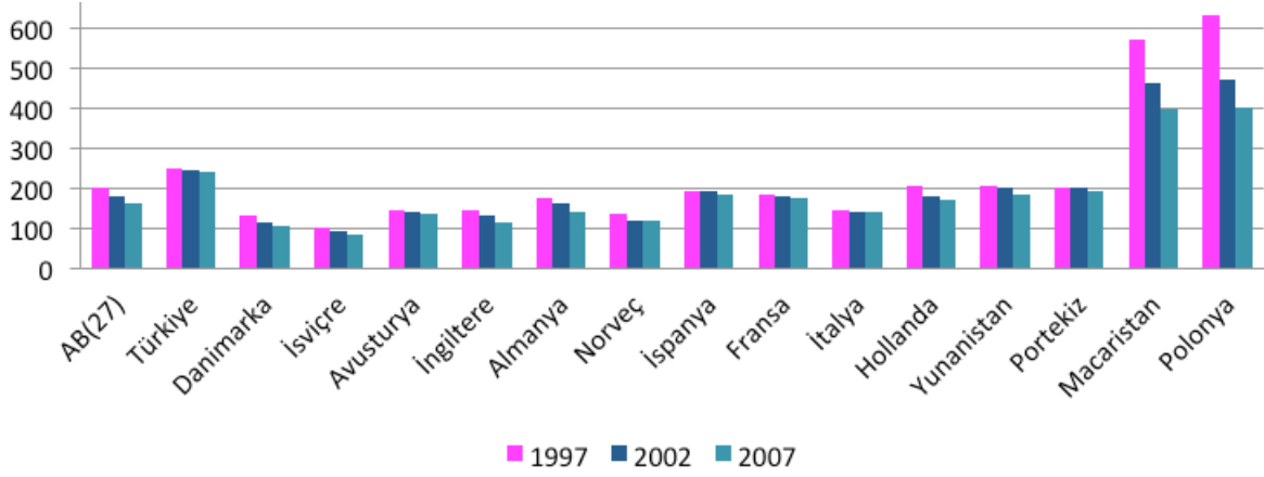
Şekil 1: Türkiye'nin Enerji Yoğunluğu Trendinin Bazı Ülkeler ile Karşılaştırılması
